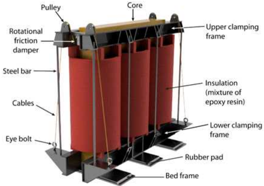
구성도
